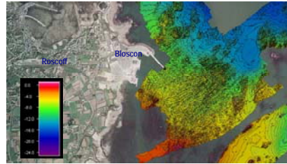
Zoom sur la bathymétrie devant le port de Blosscon (résolution de 50 cm, isobathe tous les 50 cm)
