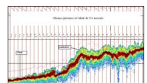
Extrait d'échogramme (ER60)
