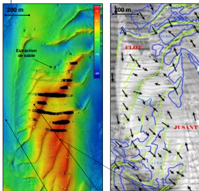
Morphodynamique du banc sableux de la Cormorandière
