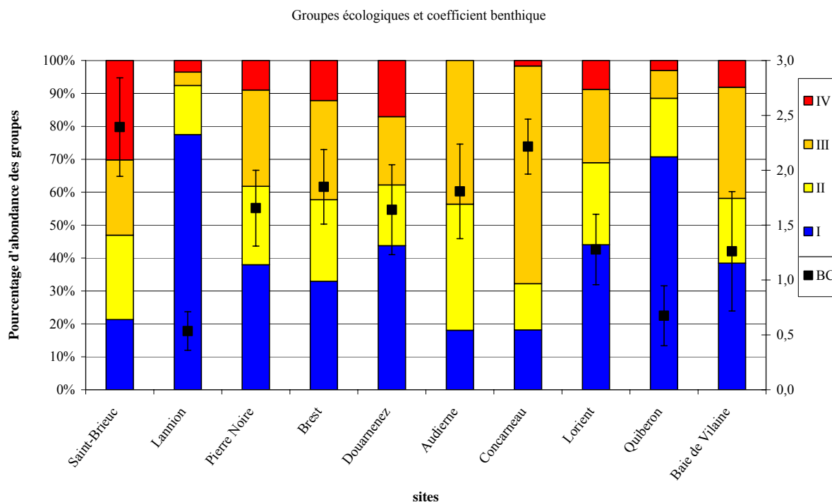
Figure 14 : Groupe écologique et coefficient benthique (BC) pour chaque site échantillonné (sites classés du nord au sud). Calculs effectués à partir des groupes de références sur le site AZTI (décembre 2007)
