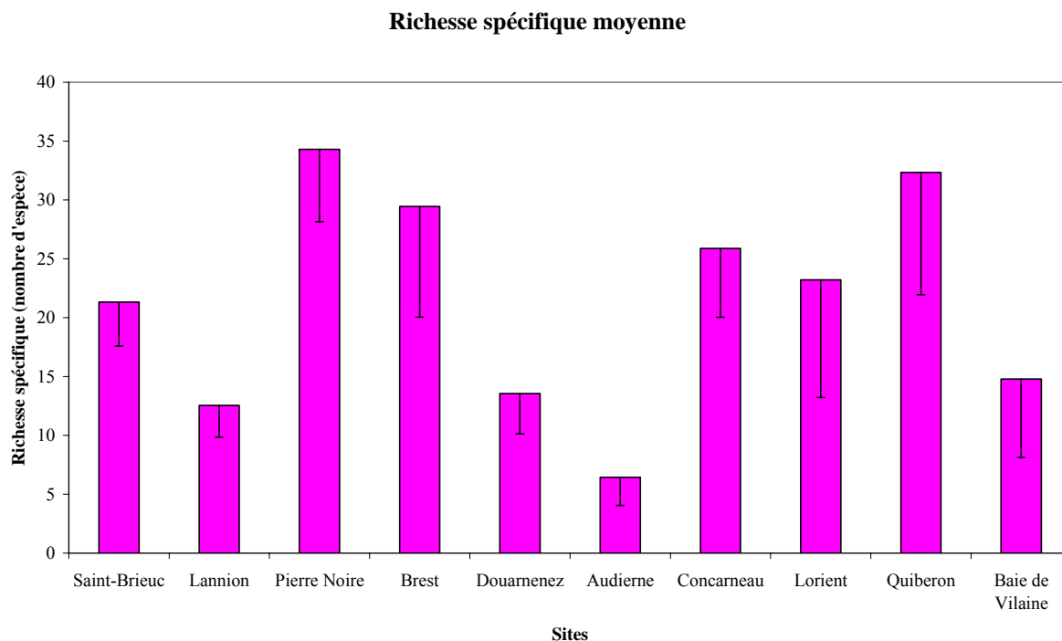
Figure 12 : Richesse spécifique moyenne (nombre moyen d'espèces par réplicat) avec l'écart-type pour chaque site échantillonné en 2009 (classé du nord au sud).
