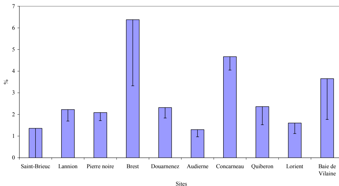
Figure 10 : Taux de matière organique moyen pour chaque site étudié en 2009 (classés du nord au sud).
