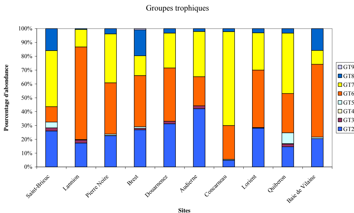
Figure 15 : Groupes trophiques en pourcentage d'abondance pour chaque site échantillonné en 2009 (sites classés du nord au sud).
