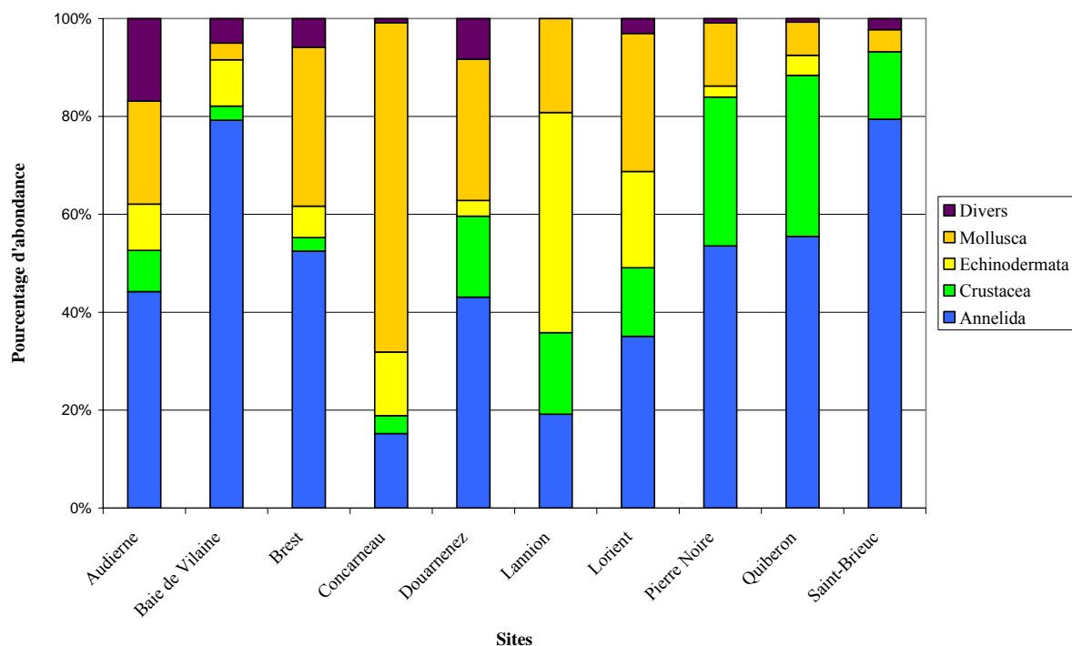
Figure 11 : Dominance des grands groupes zoologiques dans chaque site échantillonné en 2009.
