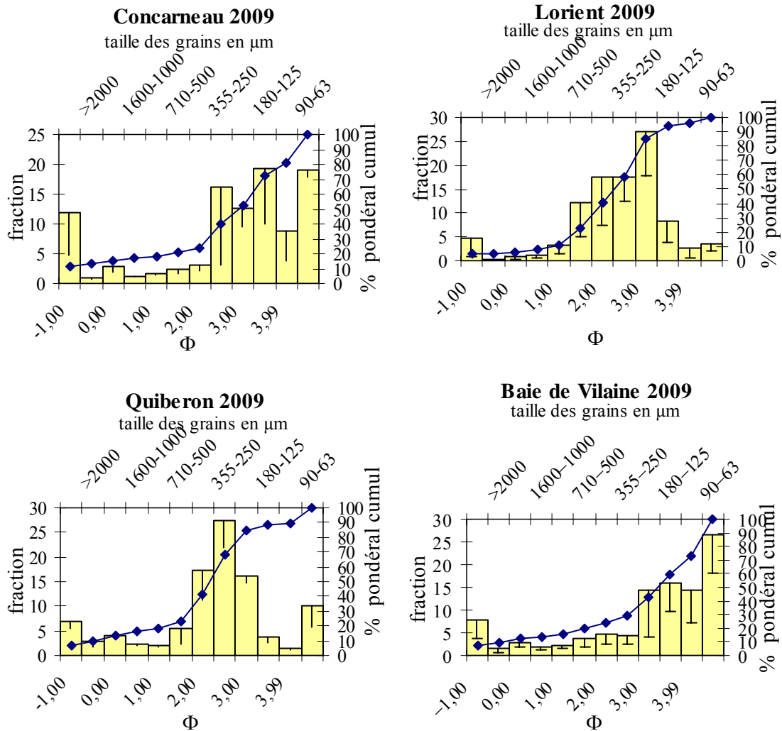
Figure 9 : Courbe granulométrique cumulée et pourcentages pondéraux des fractions granulométriques (avec écart-type) pour chaque site étudié, classé du nord au sud.
